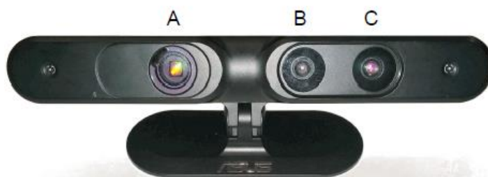
Рис. 5. Камера Asus Xtion RGB-D использует (А) инфракрасный излучатель (В) стандартную цветную камеру RGB и (С) инфракрасную камеру
