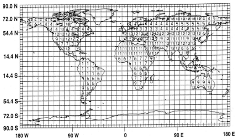
Рис.1. Использованное в модели SiB2 пространственное распределение наземных биомов по географической сетке 7.2^{\circ} \times 9.0^{\circ} [1]. Обозначения: 1 – широколиственные вечнозеленые деревья (тропический лес); 2 – широколиственные листопадные деревья; 3 – смешанные широколиственные и хвойные деревья; 4 – хвойные вечнозеленые деревья; 5 – хвойные опадающей деревья; 6 – широколиственные деревья с подлеском; 7 – луга; 8 – зеленые луга; 9 – кустарники с голой почвой; 10 – карликовые деревья и кустарники (тундра); 11 – почва без растительного покрова; 12 – сельскохозяйственные растения.
